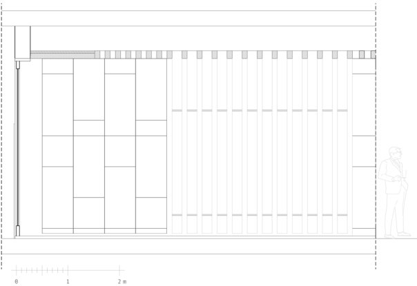
ALZADO D
