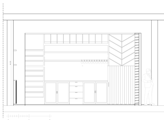
ALZADO A
